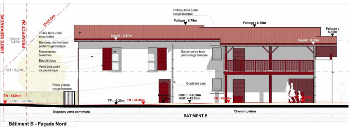
Bâtiment B - Façade Nord
