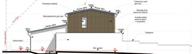
FACADE EST PROJET
