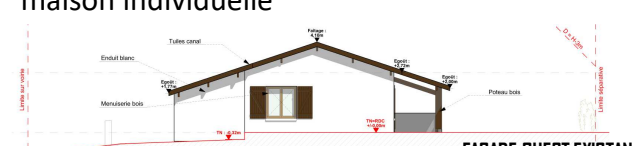
FACADE OUEST EXISTANT
