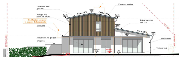
FACADE OUEST PROJET
