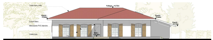
Façade Sud-Est - Existant
