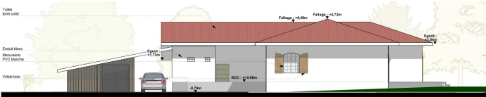
Façade Sud-Ouest - Existant
