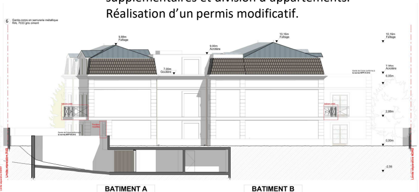
Façade Ouest
