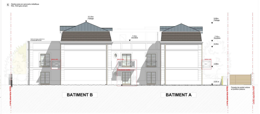
Façade Ouest
