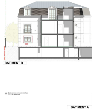
Façade Sud
